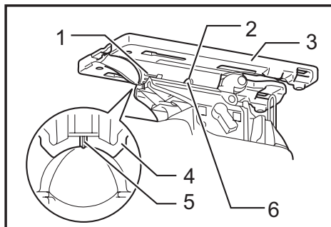
► 1. Graduation 2. Fente en biseau 3. Base 4. Carter d'engrenage 5. Encoche en V 6. Boulon
