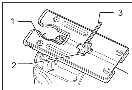
► 1. Base 2. Perno 3. Llave hexagonal
