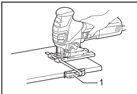
► 1. Tope lateral de corte
