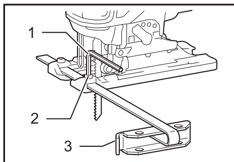
► 1. Llave hexagonal 2. Perno 3. Guía lateral
