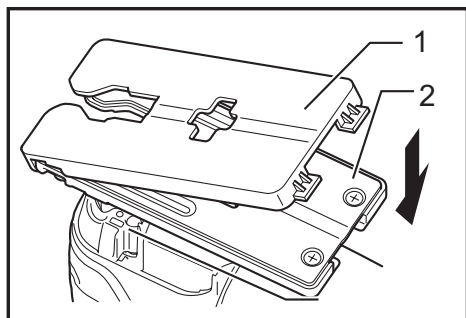
► 1. Plaque de recouvrement 2. Base
