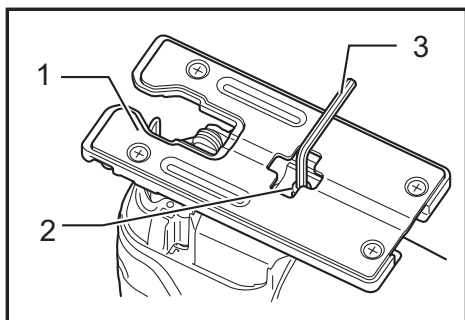
► 1. Base 2. Boulon 3. Clé hexagonale
