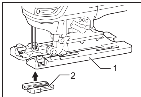
► 1. Base 2. Dispositivo antiastillado
