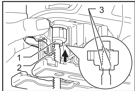
► 1. Sujetador de hoja de sierra 2. Hoja de sierra caladora 3. Protuberancias
