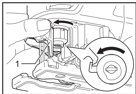
► 1. Abridor de la herramienta
