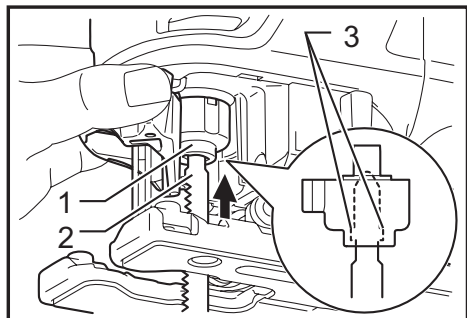
► 1. Porte-lame 2. Lame de scie sauteuse 3. Saillies
