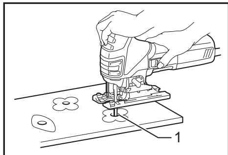
► 1. Agujero de inicio
