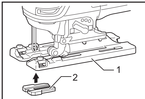
► 1. Base 2. Dispositif anti-fente
